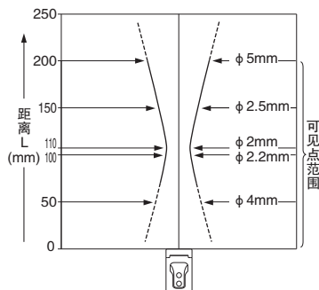
投光光束特性
