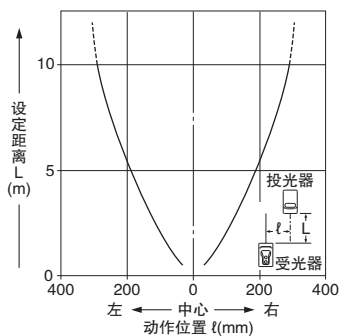
安装圆形狭缝透光罩(φ 2mm)时的平行移动特性
