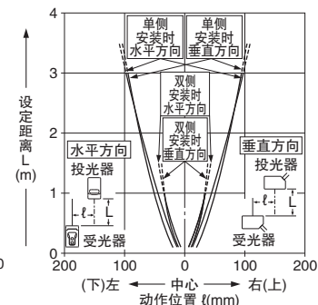
安装方形狭缝透光罩(1 × 6mm)时的平行移动特性
