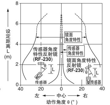
角度特性
