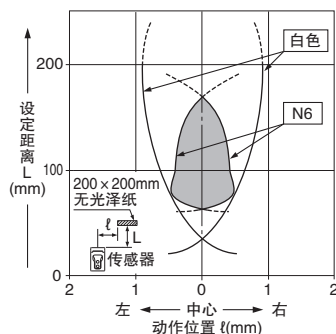
亮度和检测距离之间的相互关系
