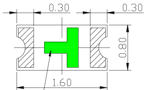
负极标志 Cathode Mark
