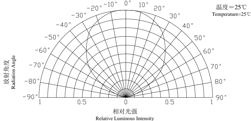
发光分布图 Radiation Diagram
